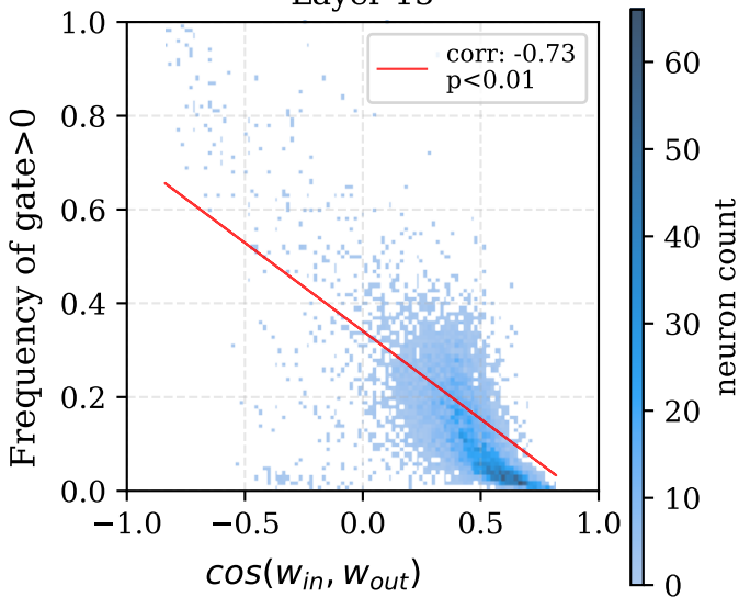
Layer 15
